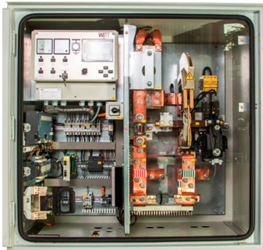
EKS1000 Außenaufstellung
